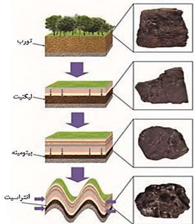
مراحل تشکیل آنتراسیت (زغال رسیده)
