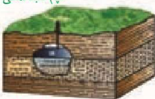
ت) ریفی (مرجانی)
