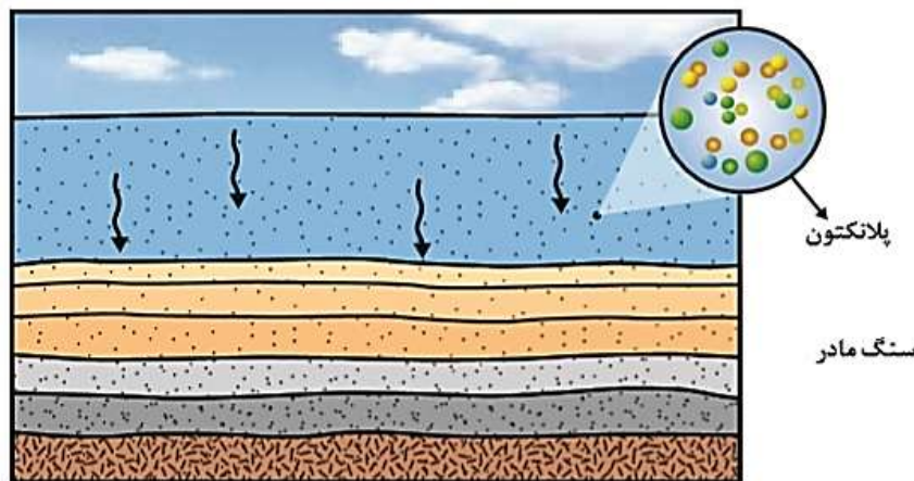
تشکیل ذخایر نفت و گاز در محیط های دریایی
