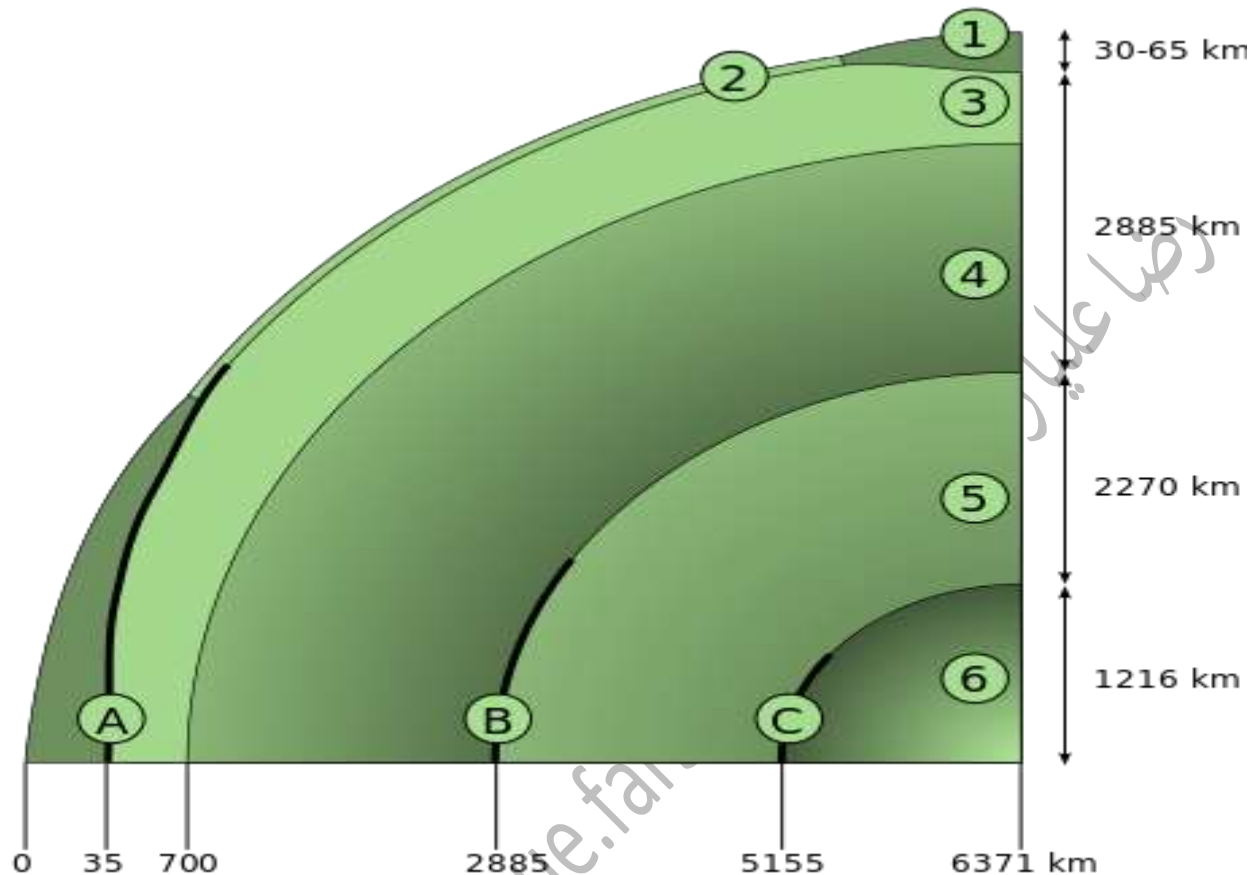
برش شماتیک درون زمین : ( Schematic section through the Earth )
